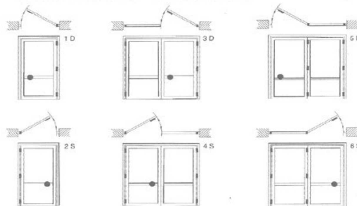
Schemi di apertura - Vista dall'interno
